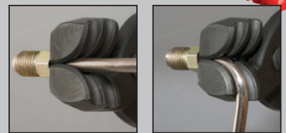
Bremsrohrzange
